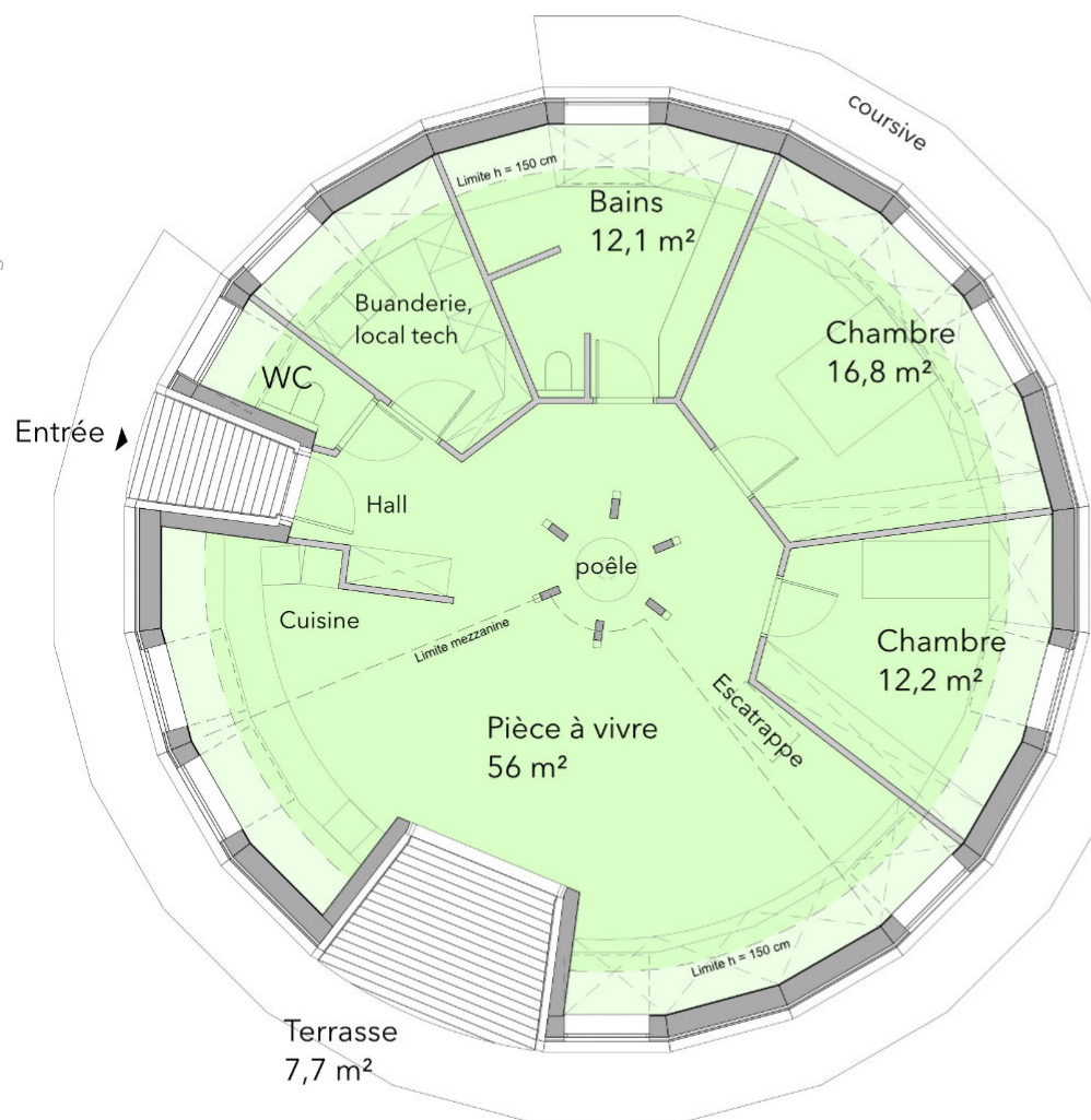
Rez-de-chaussée
