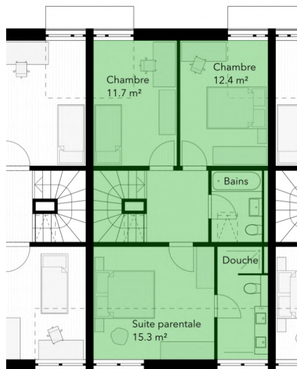
Étage
