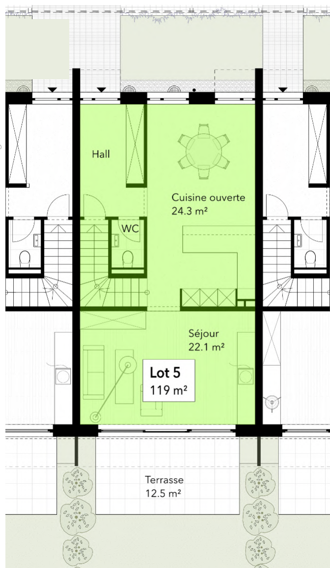
Rez-de-Chaussée
